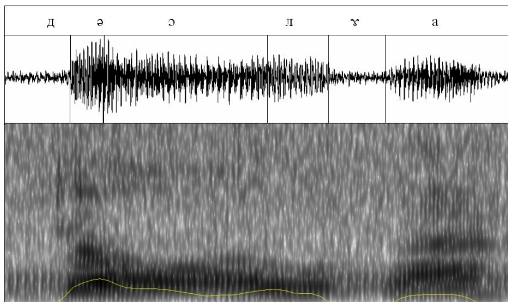
Рис. 2.25. Осциллограмма, спектрограмма и огибающая интенсивности формы д[\overset{\circ}{э}]лго (с. Новосёлки Рыбновского р-на Рязанской обл.)
