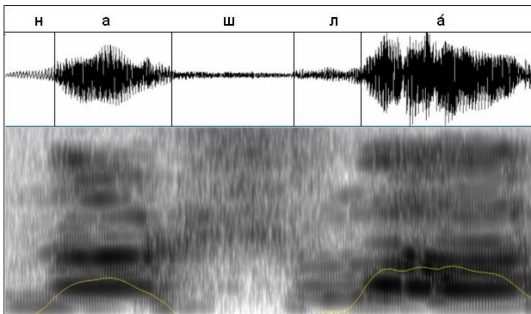
Рис. 1.35. Осциллограмма, спектрограмма и огибающая интенсивности формы нашlá (д. Желачек, о-в Пийриссаар, Эстония)
