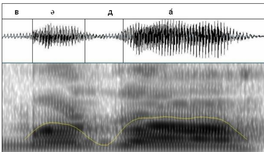
Рис. 1.36. Осциллограмма, спектрограмма и огибающая интенсивности формы водá (д. Желачек, о-в Пийриссаар, Эстония)
