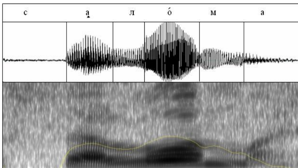
Рис. 4.5. Осциллограмма, спектрограмма и огибающая интенсивности формы солóма (с. Берёзовка Ивнянского р-на Белгородской обл.)
