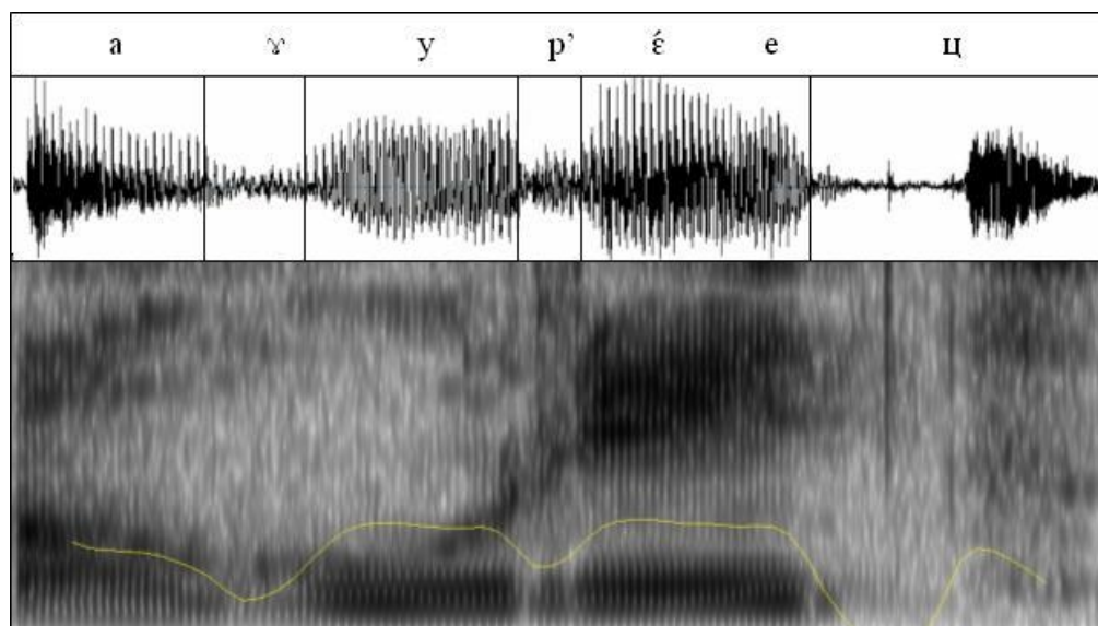
Рис. 2.21. Осциллограмма, спектрограмма и огибающая интенсивности формы огур[’έε]ц (с. Солдатское Старооскольского р-на Белгородской обл.)
