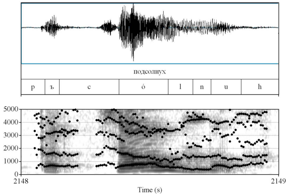
Рисунок 4.6. Осциллограмма и спектрограмма словоформы [пъцѝлнух] – подсолнух
