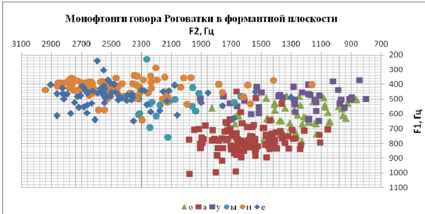
Рис. 3.2. Монофтонги говора Роговатки перед твёрдыми согласными в пространстве F1 и F2
