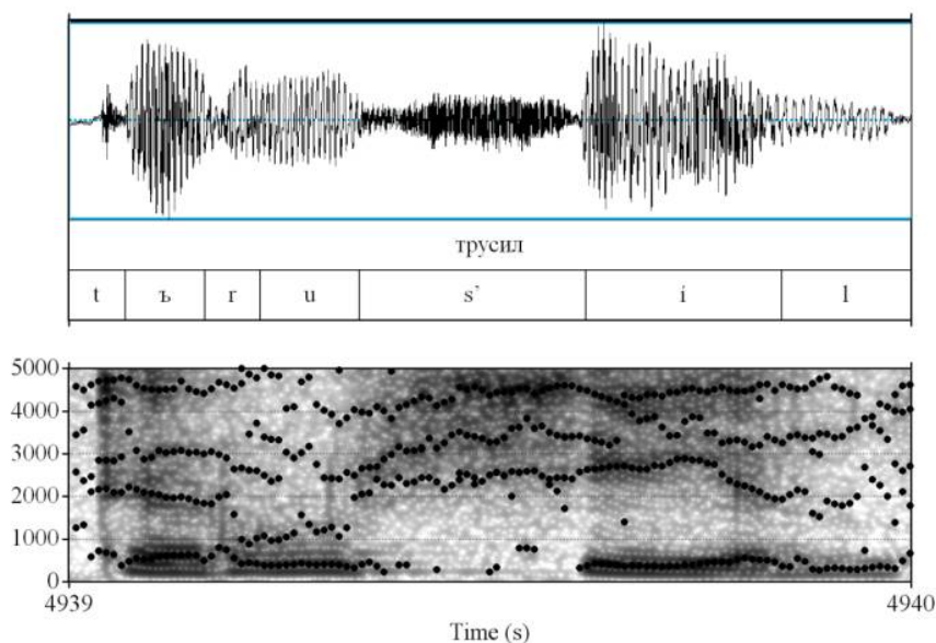
Рисунок 3.21. Осциллограмма и спектрограмма словоформы [трус'і л] – трусил
