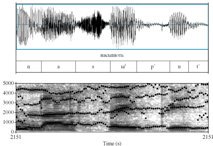
Рисунок 3.17. Осциллограмма и спектрограмма словоформы [насып'ут'] – насыпютъ
