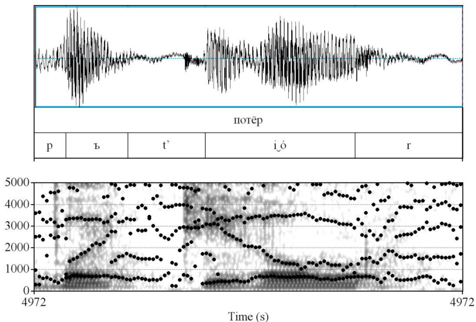
Рисунок 3.45. Осциллограмма и спектрограмма словоформы [пѣт'иѡр] – потёр
