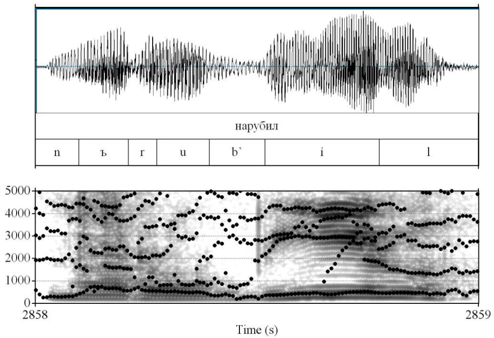
Рисунок 3.25. Осциллограмма и спектрограмма словоформы [куп'и ла] – купила
