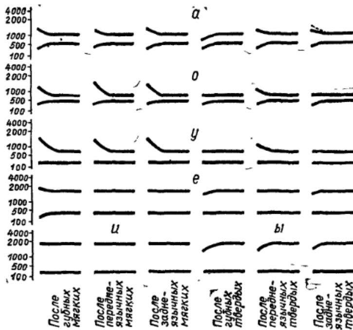
Рис. 3.8. Схематические изображения изменения F1 и F2 русских гласных после разных согласных (по [Бондарко 1977: 65])
