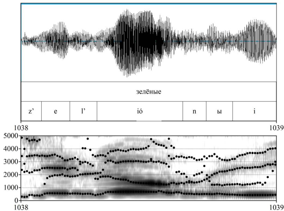
Рисунок 4.14. Осциллограмма и спектрограмма словоформы [з'ел'и́оны] – зелёные
