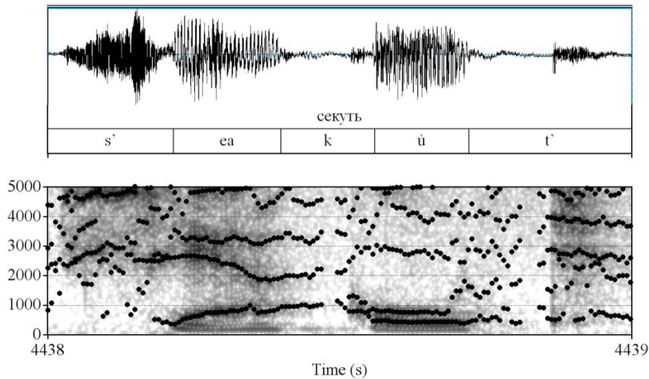
Рисунок 4.8. Осциллограмма и спектрограмма словоформы [с'еакút'] – секут
