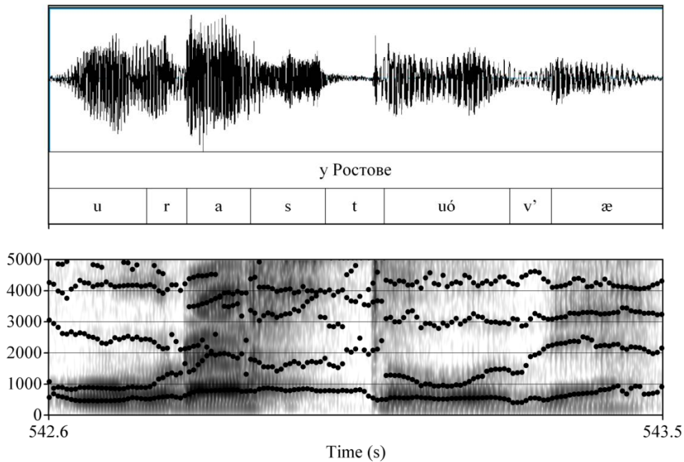
Рисунок 3.42. Осциллограмма и спектрограмма словоформы [у Расту́б'а] – у Ростове
