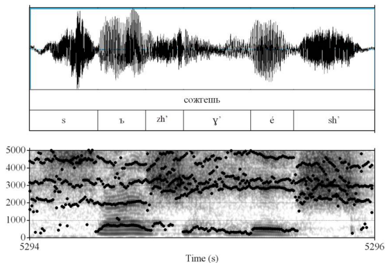
Рисунок 4.5. Осциллограмма и спектрограмма словоформы [с'ъж'у'эш'] – сожгешь
